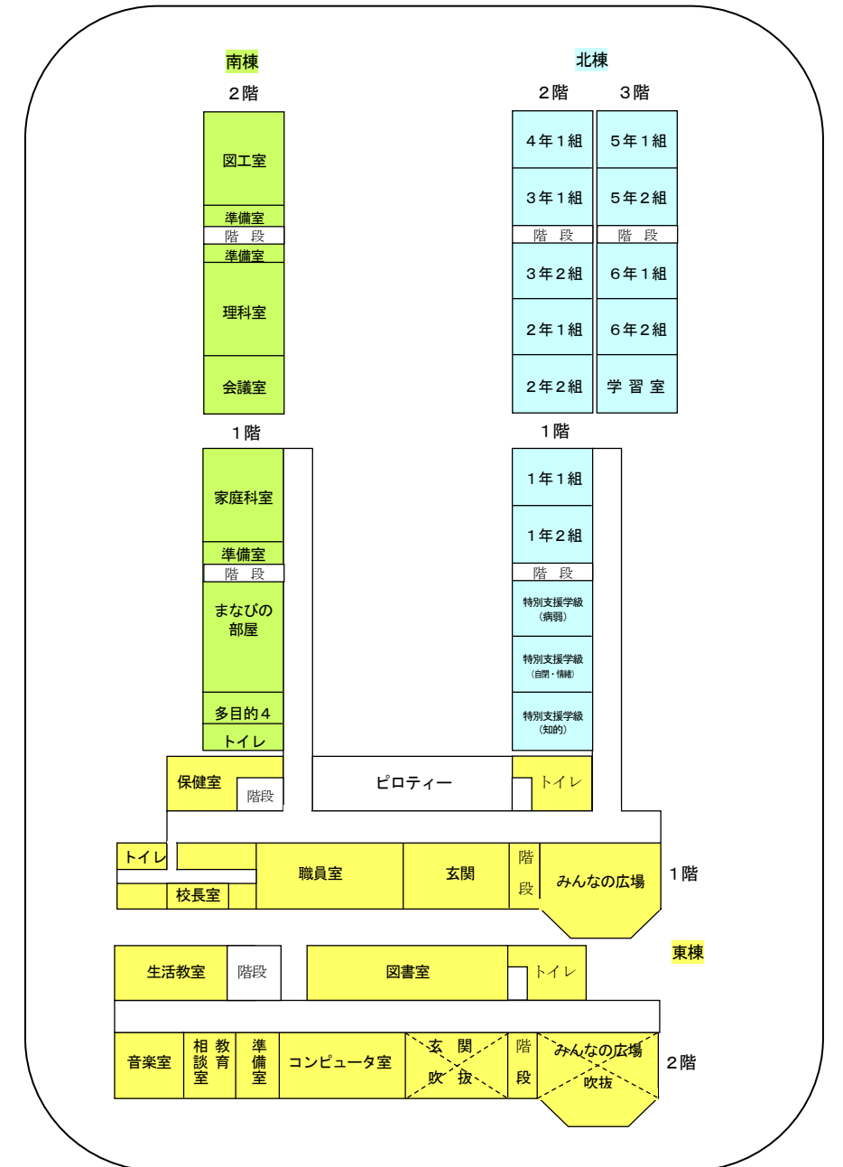
校舎配置図
